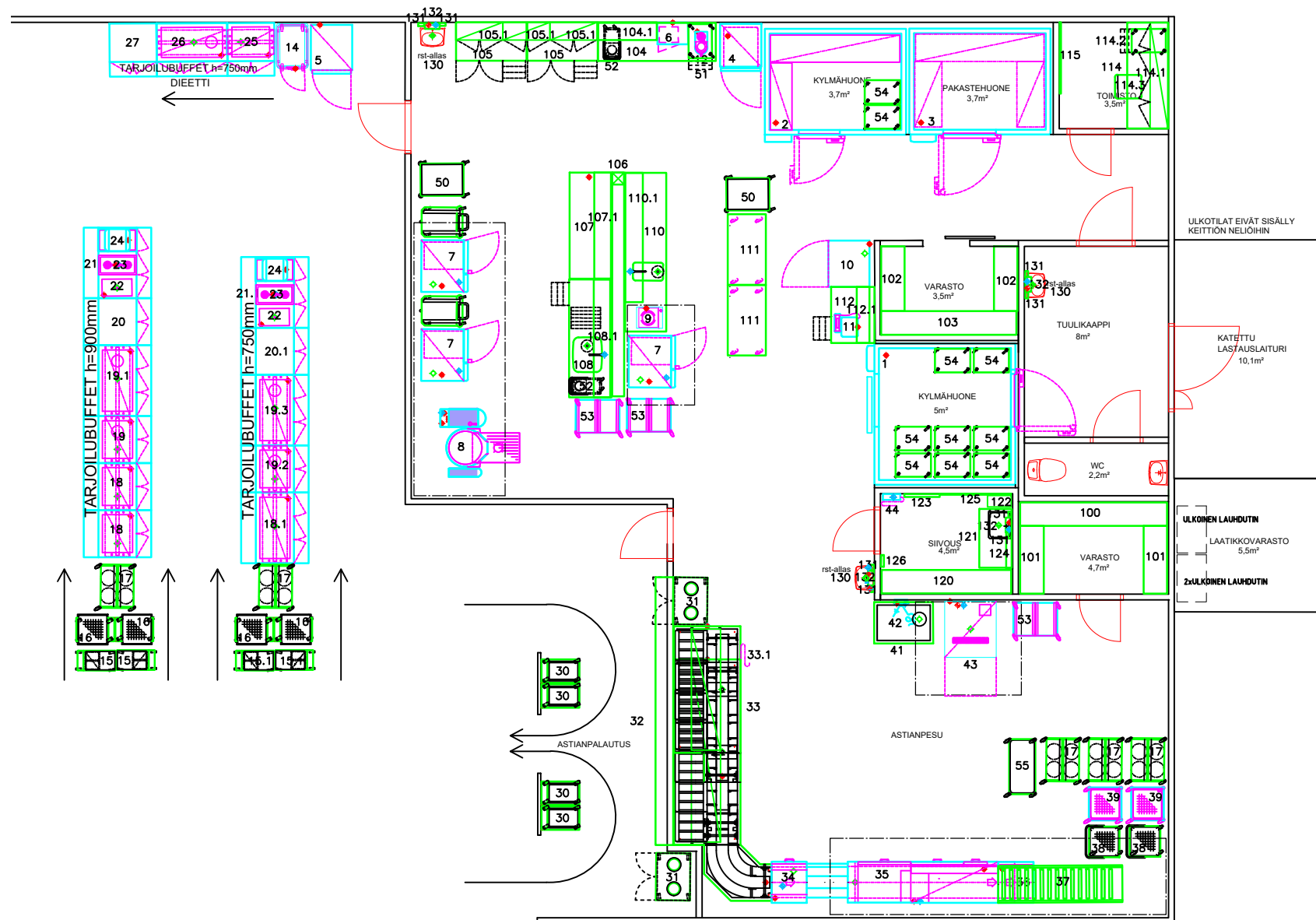
PIRKANMAAN VOIMIA PALVELUKEITTIÖ KOULU 500 ANNOSTA SUUNNITELMALUONNOS 163 m2 A3/1:100
