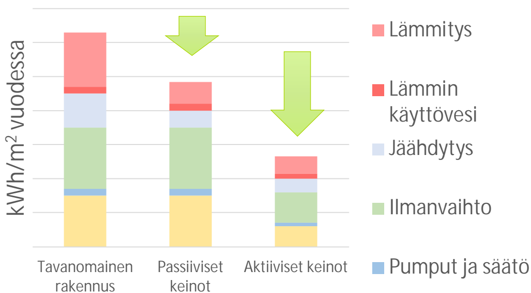
KUVA 2: PASSIIIVISTEN JA AKTIIVISTEN KEINOJEN VAIKUTUKSET RAKENNUKSEN ENERGIANKULUTUKSEEN.
