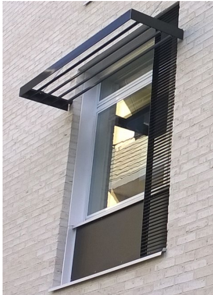
Kuva 5. Koukkuniemen Impivaaran aurinkosuojus, joka samalla estää uloimman ikkunalasin huurtumisen syksyllä tietyissä sääolosuhteissa.
